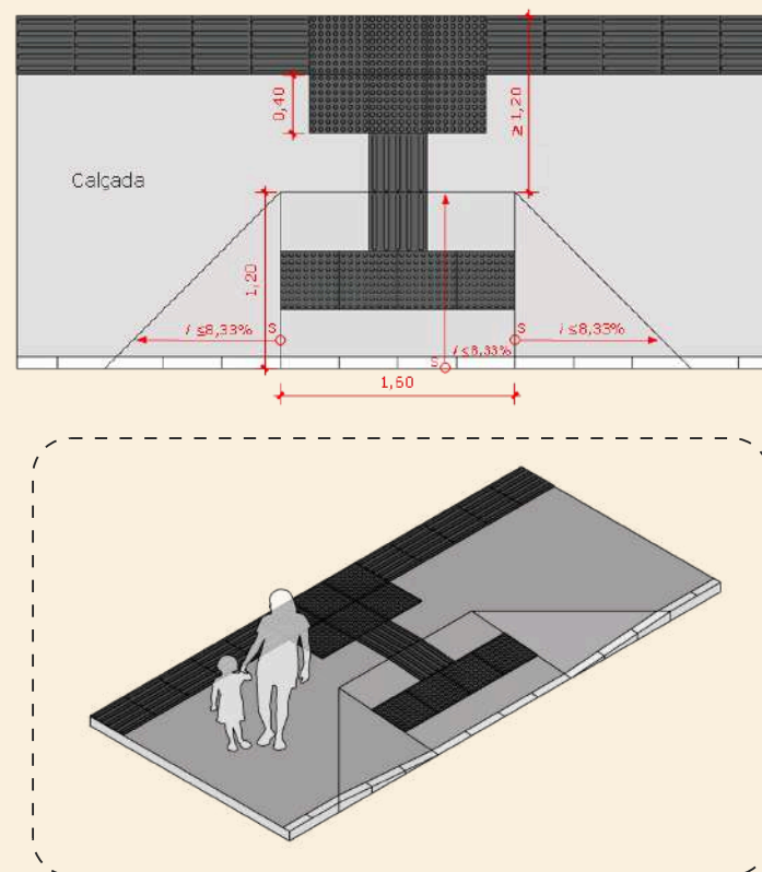
Rebaixamento calçada de piso de 40cm - Vista superior e perspectiva
