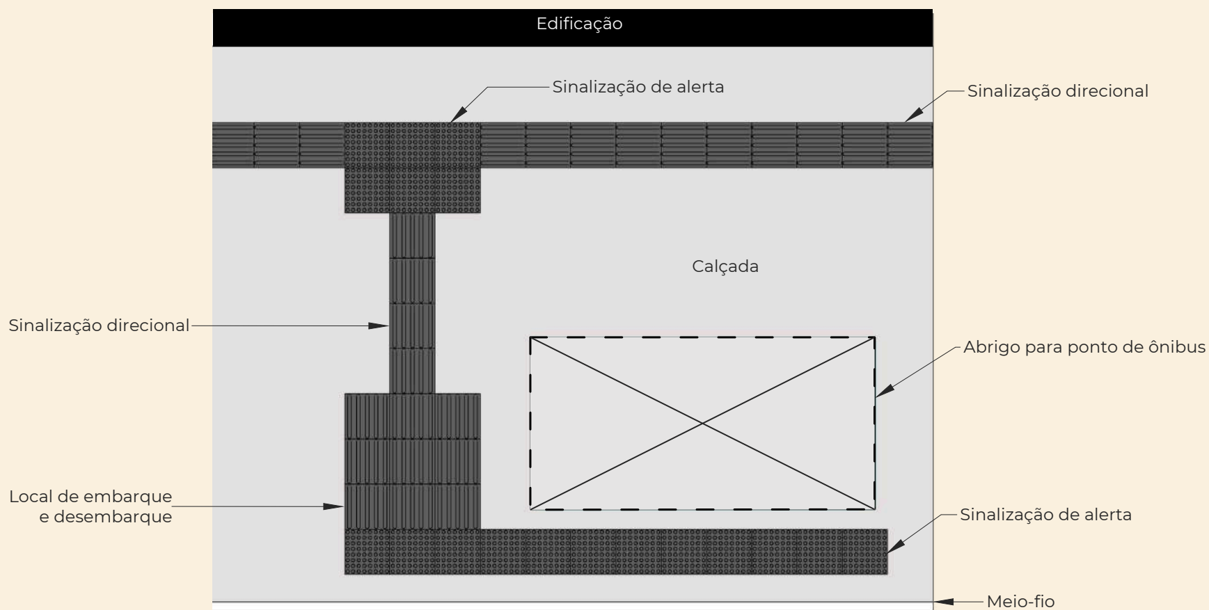
Ponto de ônibus em calçada com sinalização tátil direcional - Vista superior
