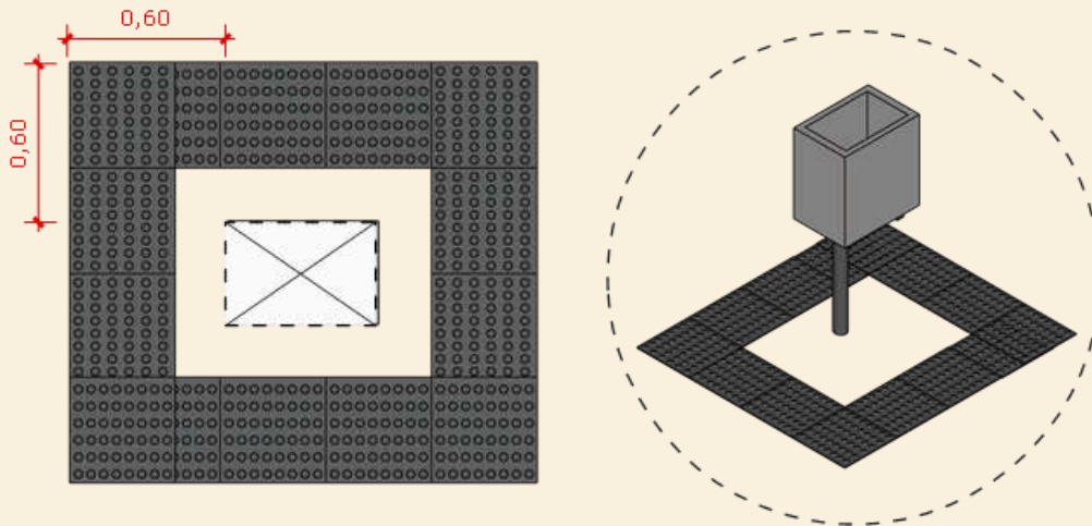
Piso tátil em objeto autoportante
