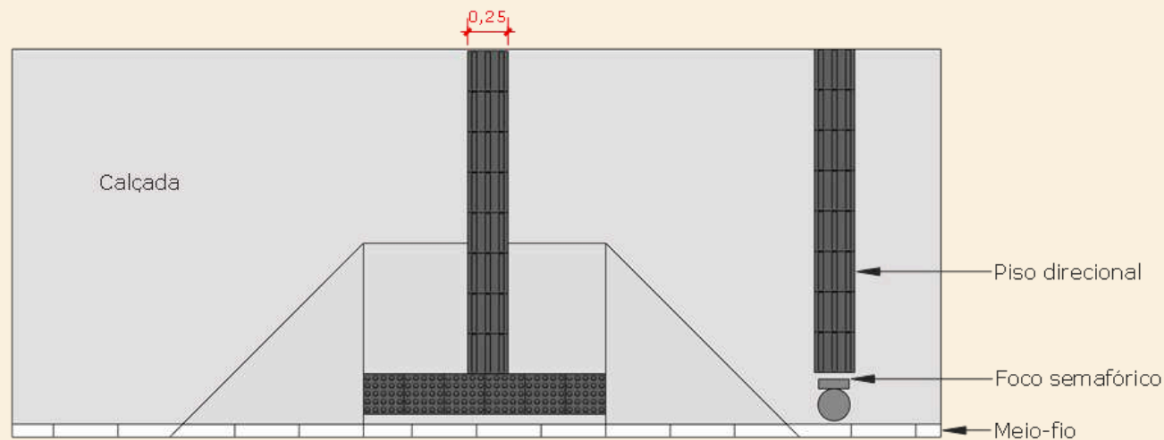
Travessia com foco semafórico em calçada com sinalização de 25cm - Vista superior
