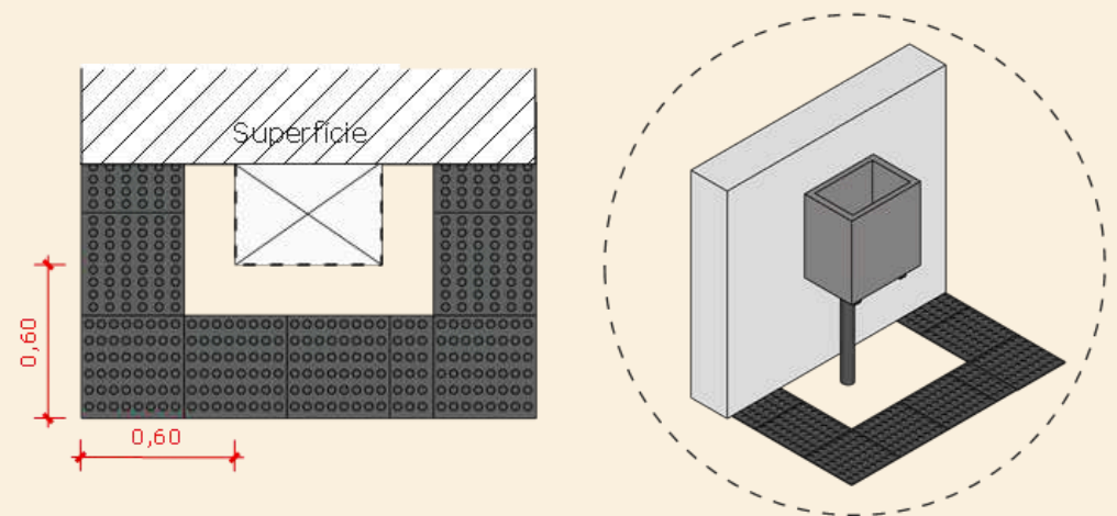
Piso tátil em objeto fixado em superfície vertical
