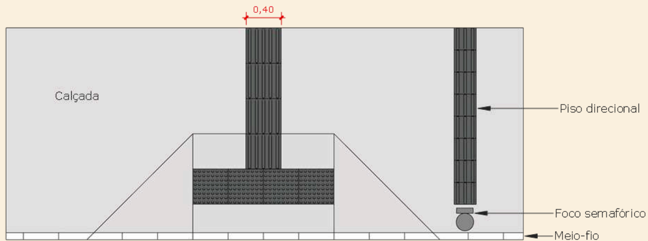
Travessia com foco semafórico em calçada com sinalização de 40cm - Vista superior
