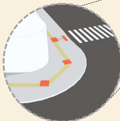
DETALHE MUDANÇA DE DIREÇÃO DO PISO TÁTIL
