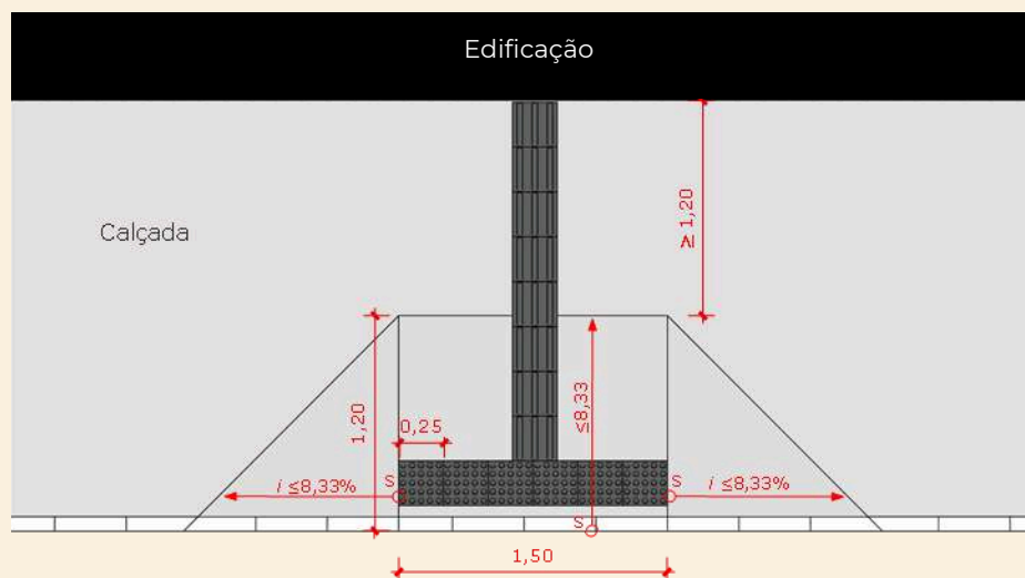
Rebaixamento calçada de piso de 25cm sem continuidade- Vista superior
