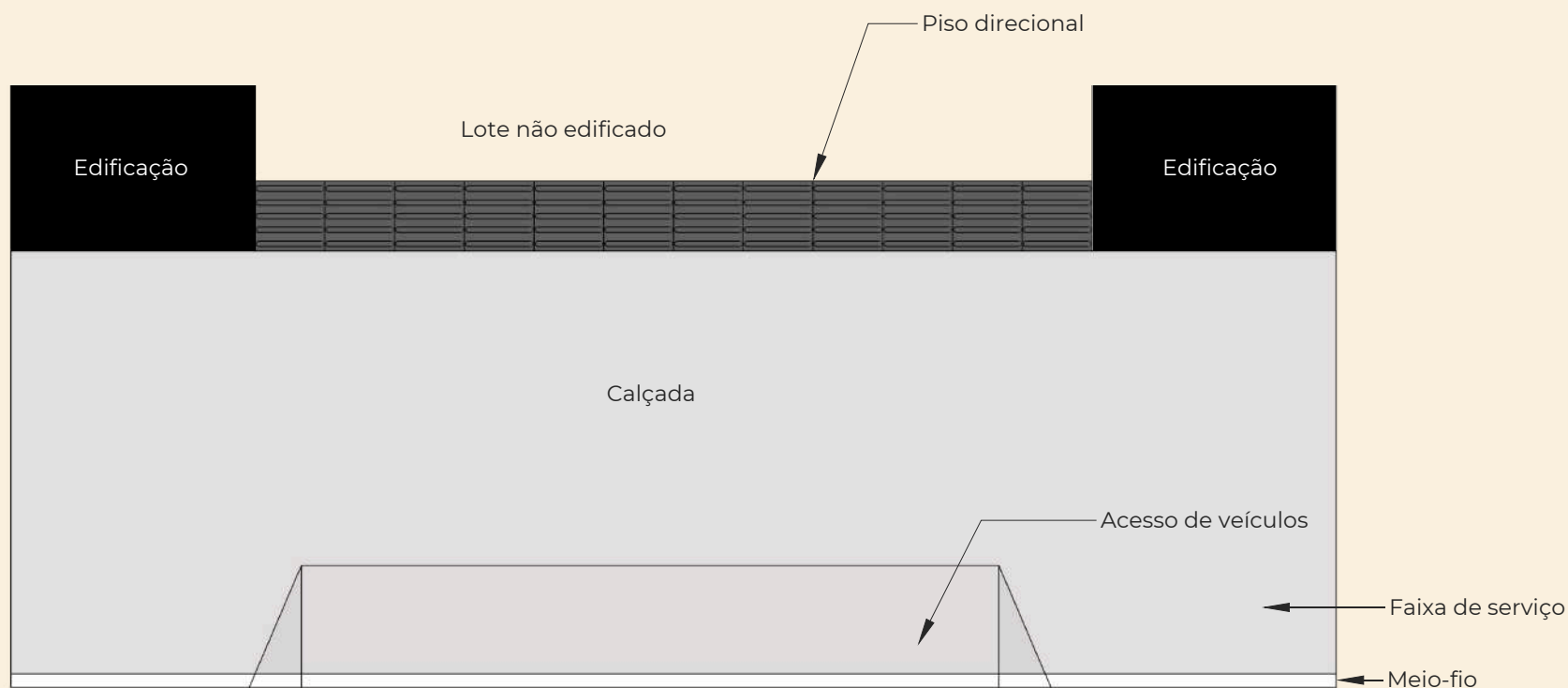
Entrada de veículos em lote não edificado - Vista superior
