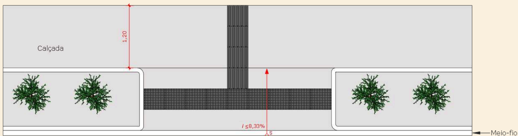
Rebaixamento calçada entre canteiros - Vista superior
