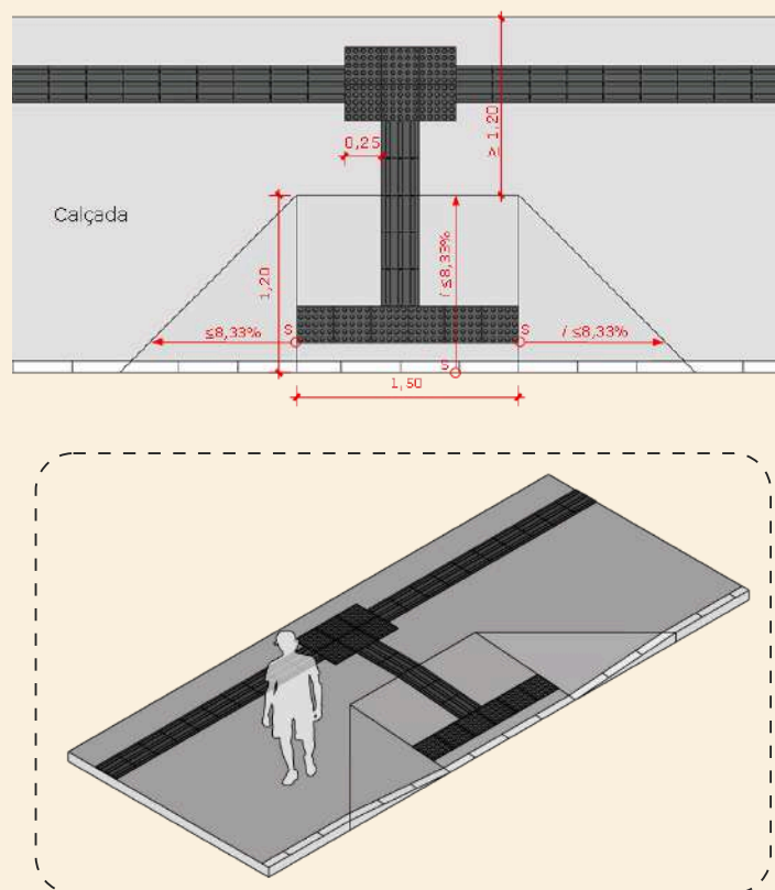
Rebaixamento calçada de piso de 25cm - Vista superior e perspectiva
