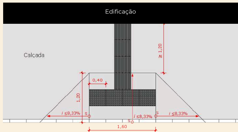
Rebaixamento calçada de piso de 40cm sem continuidade - Vista superior
